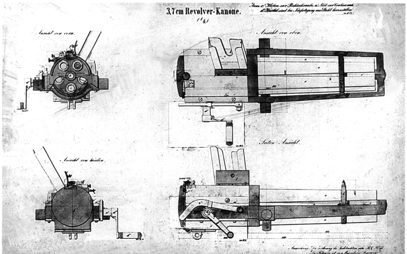
Für die Nahabwehr in den Festungen wurde 1884 die 3,7-cm Revolverkanone eingeführt. Eine sächsische Besonderheit ist, daß die Kanone für den Einsatz auf der Festung Königstein/Sachsen auf eine aptierte Lafette der 9-cm Kanone montiert wurde.
