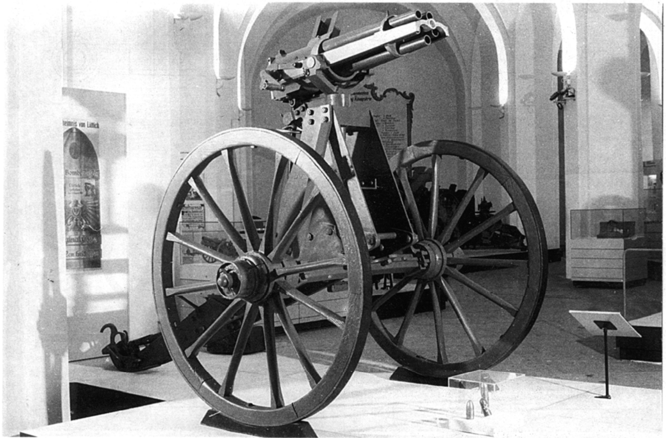
Für die Nahabwehr in den Festungen wurde 1884 die 3,7-cm Revolverkanone eingeführt. Eine sächsische Besonderheit ist, daß die Kanone für den Einsatz auf der Festung Königstein/Sachsen auf eine aptierte Lafette der 9-cm Kanone montiert wurde.
